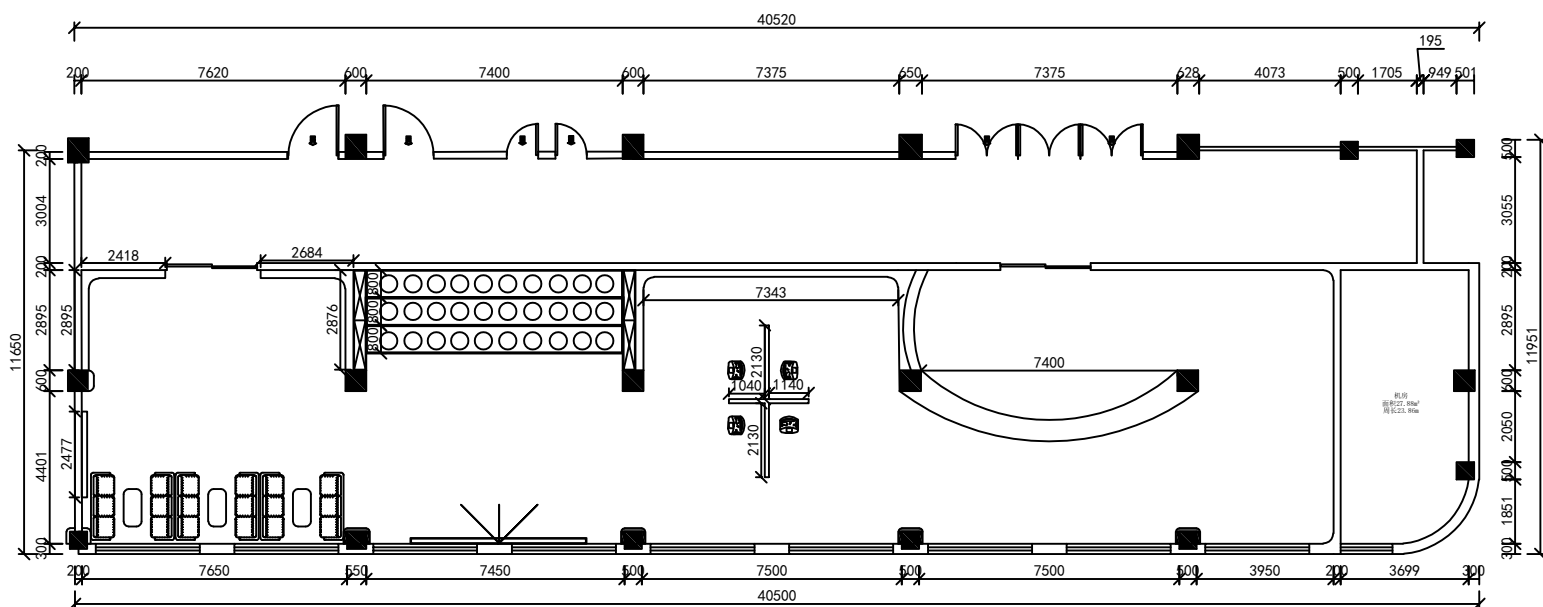
平面布局图
